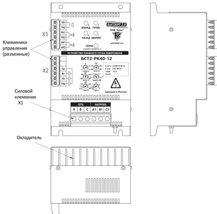
Рисунок 1 - Внешний вид пускателя БСТ2-РК40-12 (см. также Приложение А)
